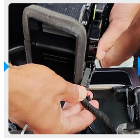
8. 将一分二电源线另一端与出风口电源线接口相连
