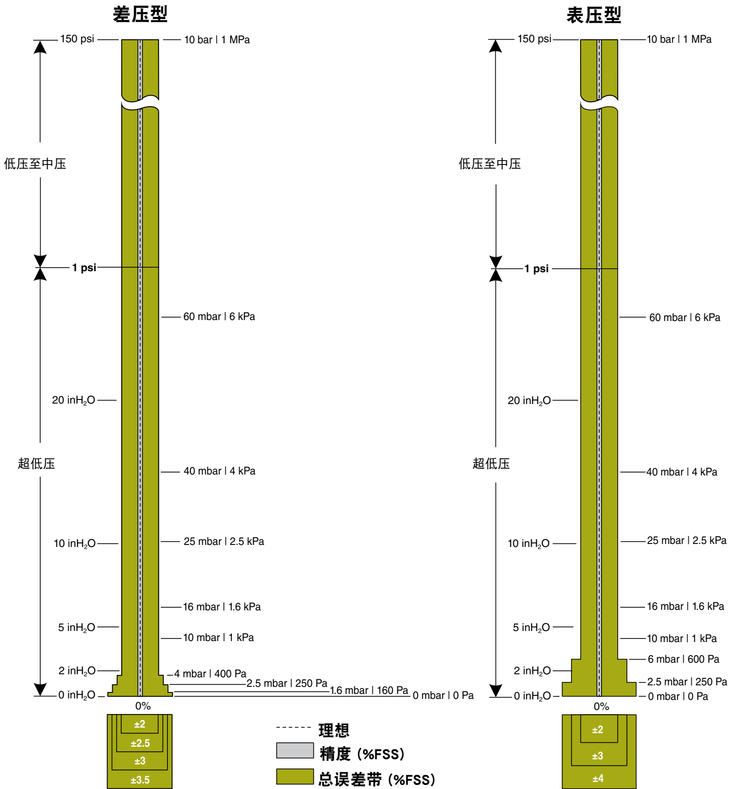
图 3. 满量程压力范围的总误差带值
