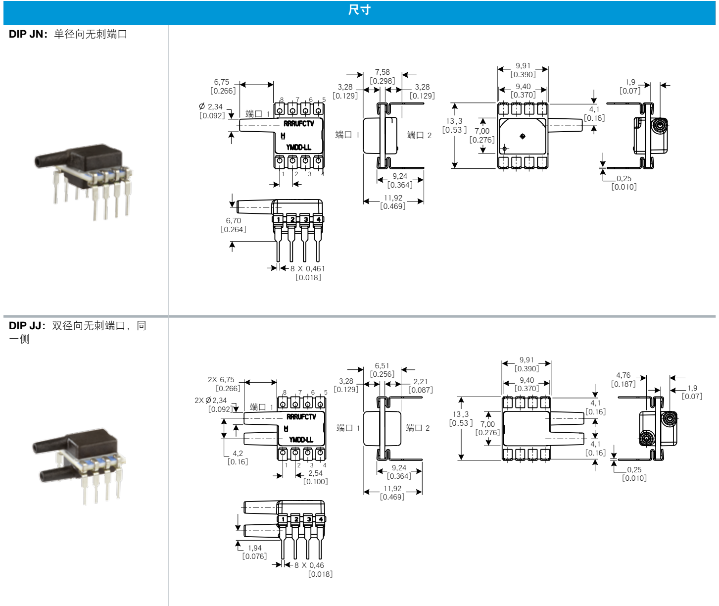
图 6. DIP 封装尺寸图 (续)
