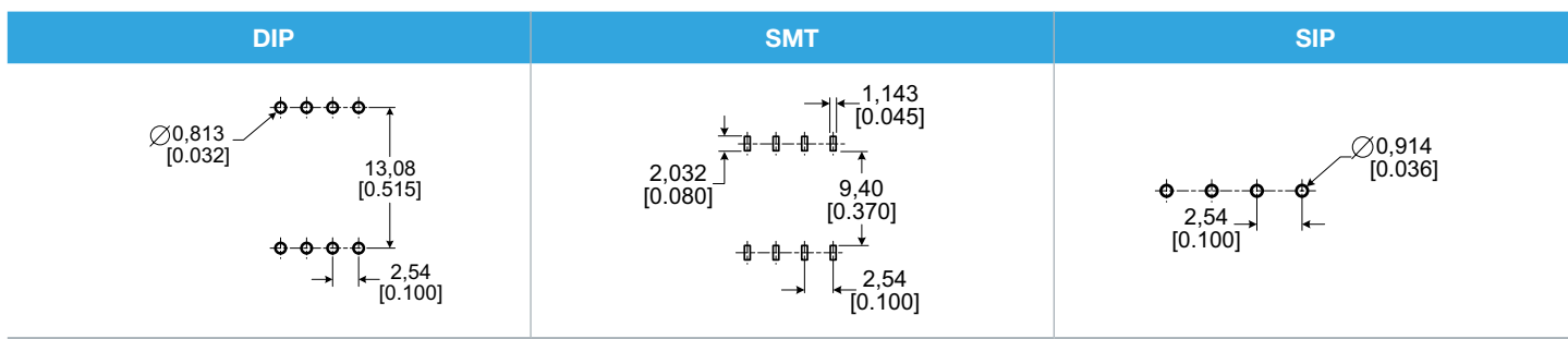
图 9.推荐 PCB 焊盘布局
