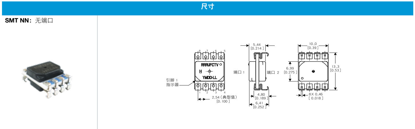
图 7. SMT 封装尺寸图 (仅供参考: mm [in.])
