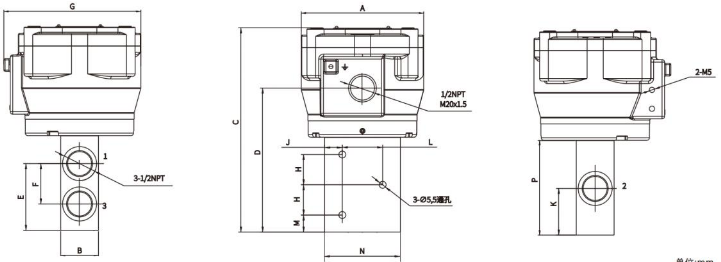
管接式阀体配EP线圈外形尺寸表
