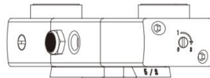
双电控NAMUR式阀体
