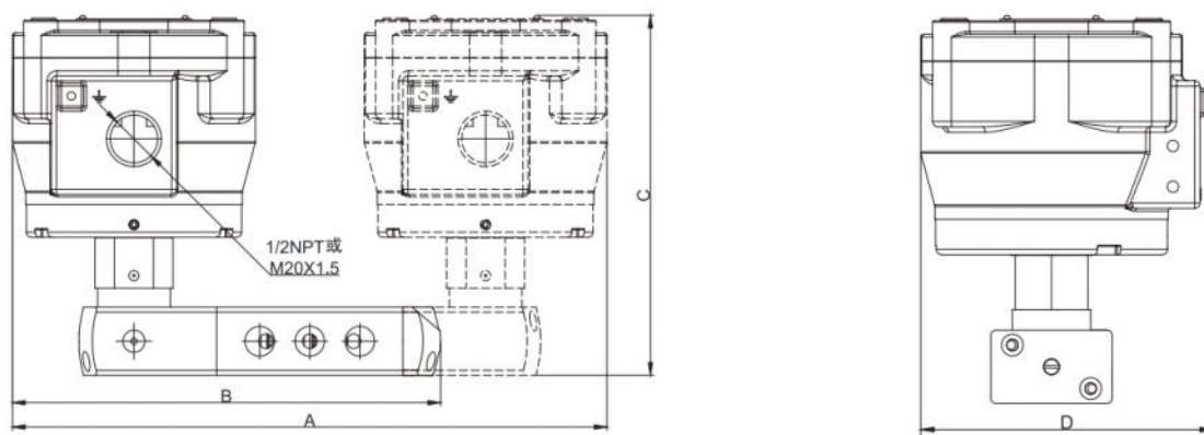
EP线圈配P52X0H/G系列管接式1/4阀体外形尺寸图
