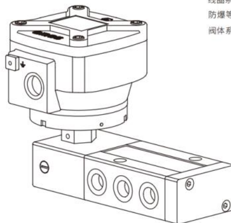
管接式1/2阀体配EPXX系列单电控简图
