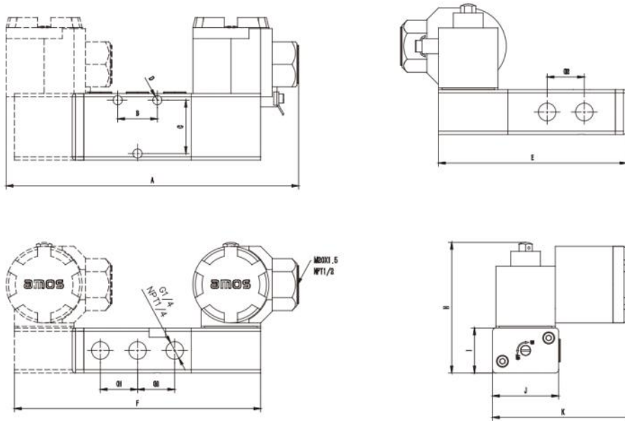
P5220H/G系列管接式1/4阀体外形尺寸图
