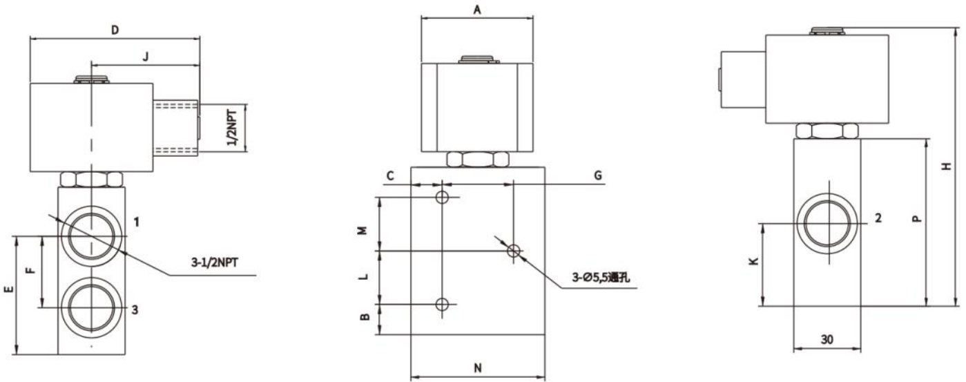
管接式阀体配ES线圈外形尺寸表
