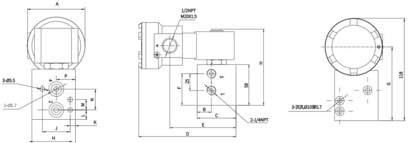
NAMUR式阀体配EB线圈外形尺寸表
