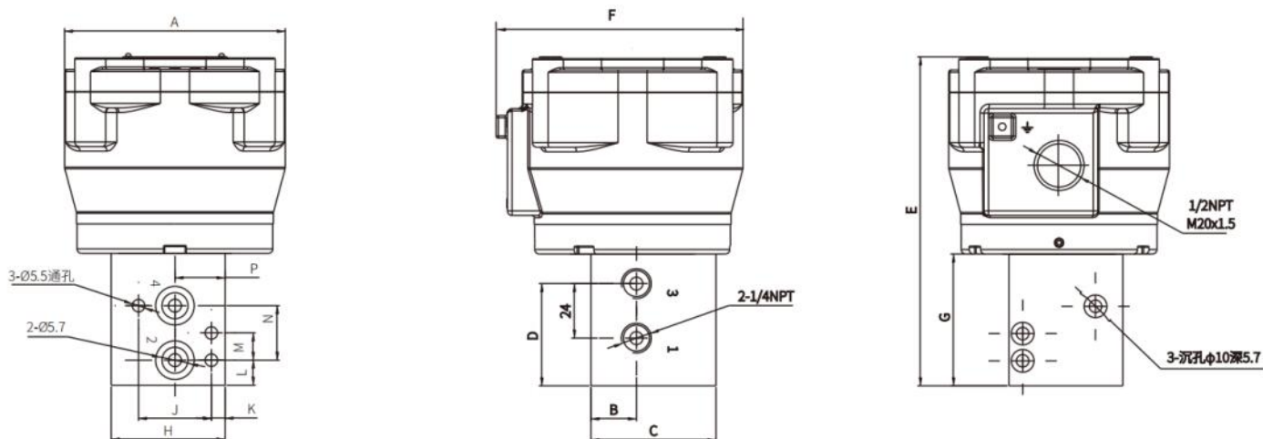
NAMUR式1/4阀体配EP线圈外形尺寸图
