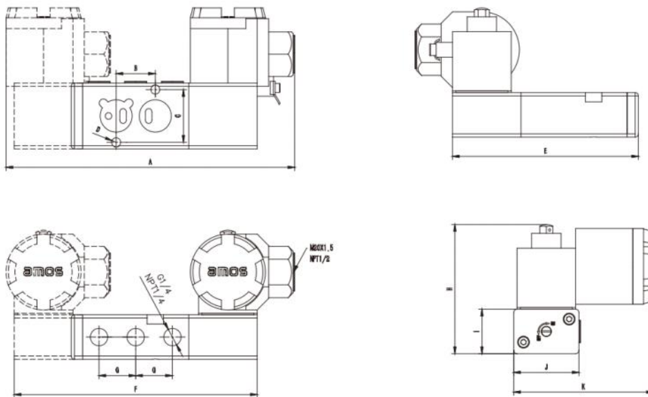
P5220H/G系列NAMUR式数据表
