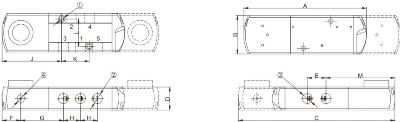
P52X0H/G系列管接式1/4阀体外形尺寸图
