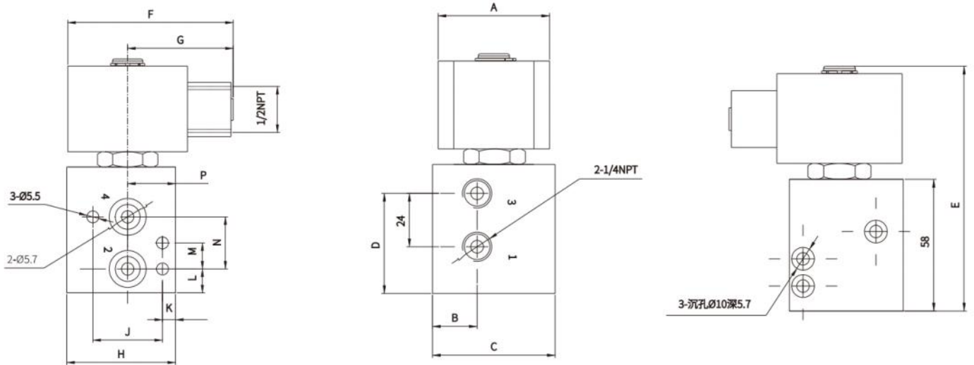
NAMUR式1/4阀体配ES线圈外形尺寸图
