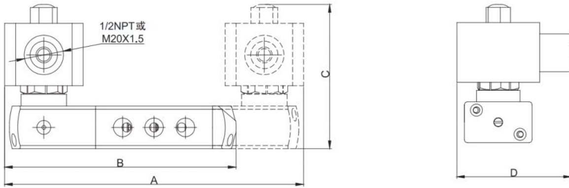
ES、AS线圈配P52X0H/G系列管接式1/4阀体外形尺寸图
