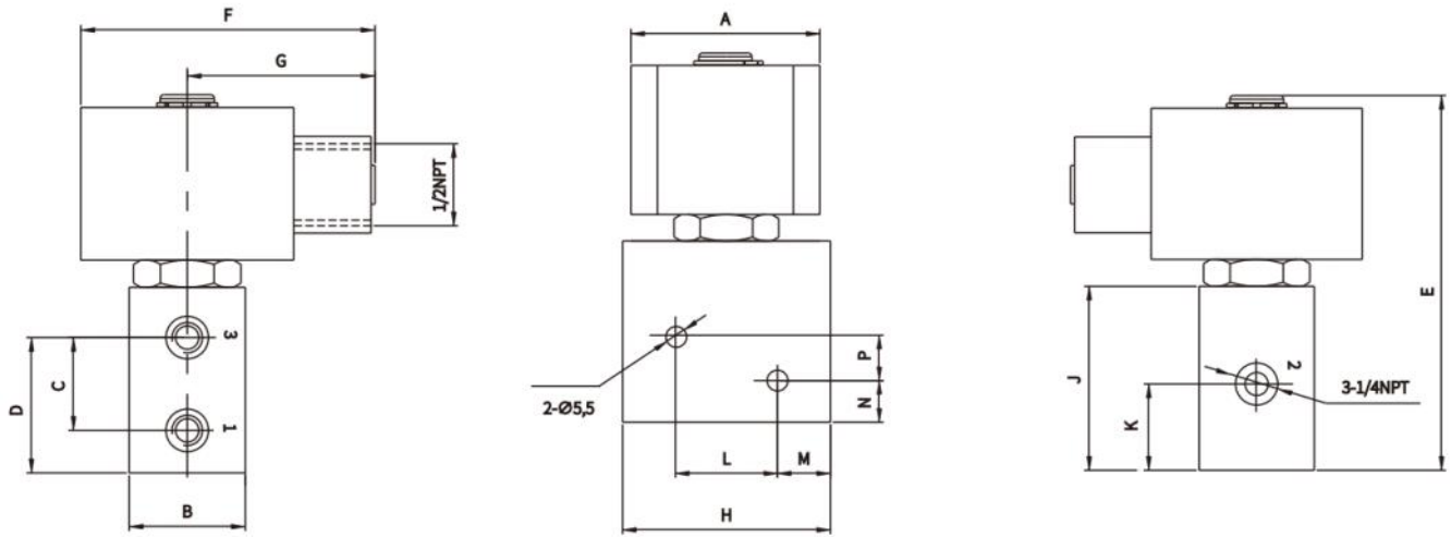
管接式1/4阀体配ES线圈外形尺寸图
