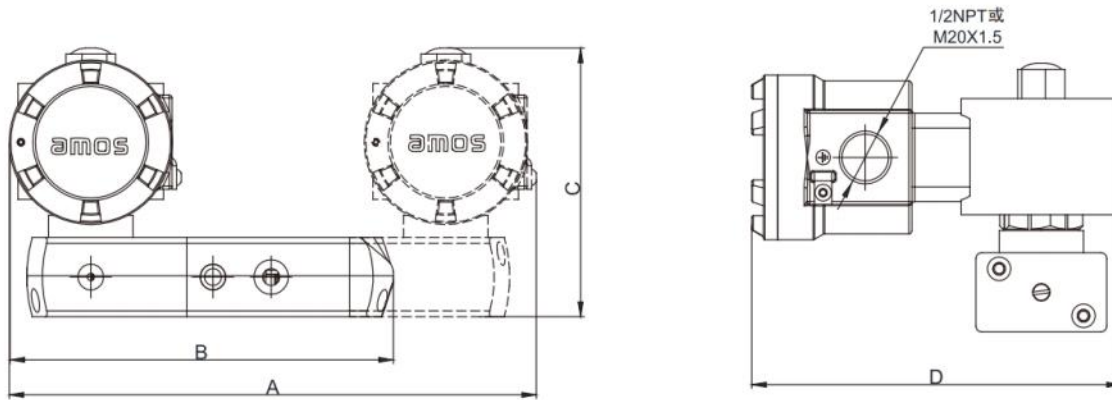
EB、EA、AB线圈配P52X0H/G系列NAMUR式1/4阀体外形尺寸图
