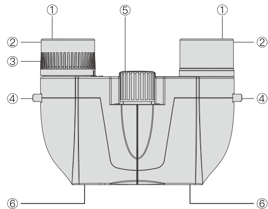
① 目镜 ② 眼罩 ③ 视度手轮 ④ 背带孔 ⑤ 调焦手轮 ⑥ 物镜
