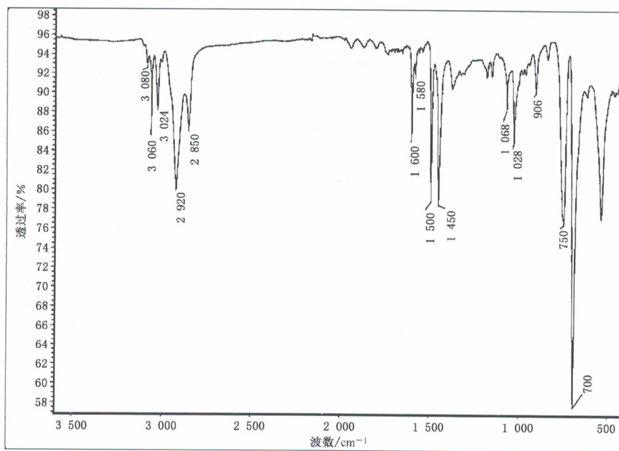
图 A.1 典型聚苯乙烯(PS)参考透射红外光谱图
