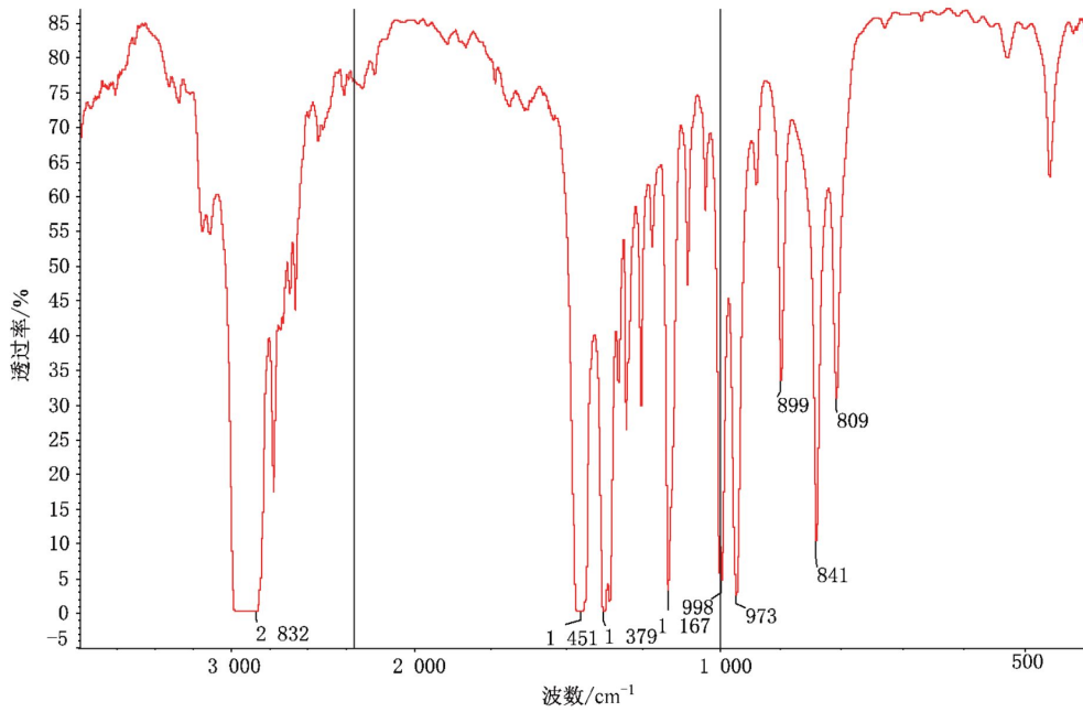
图 A.1 典型丙烯均聚物(PP-H)参考透射红外光谱图
