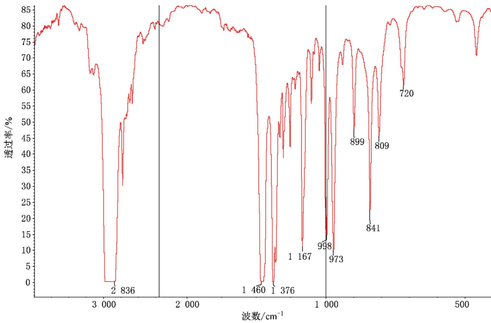
图 A.2 典型丙烯耐冲击共聚物(PP-B)参考透射红外光谱图
