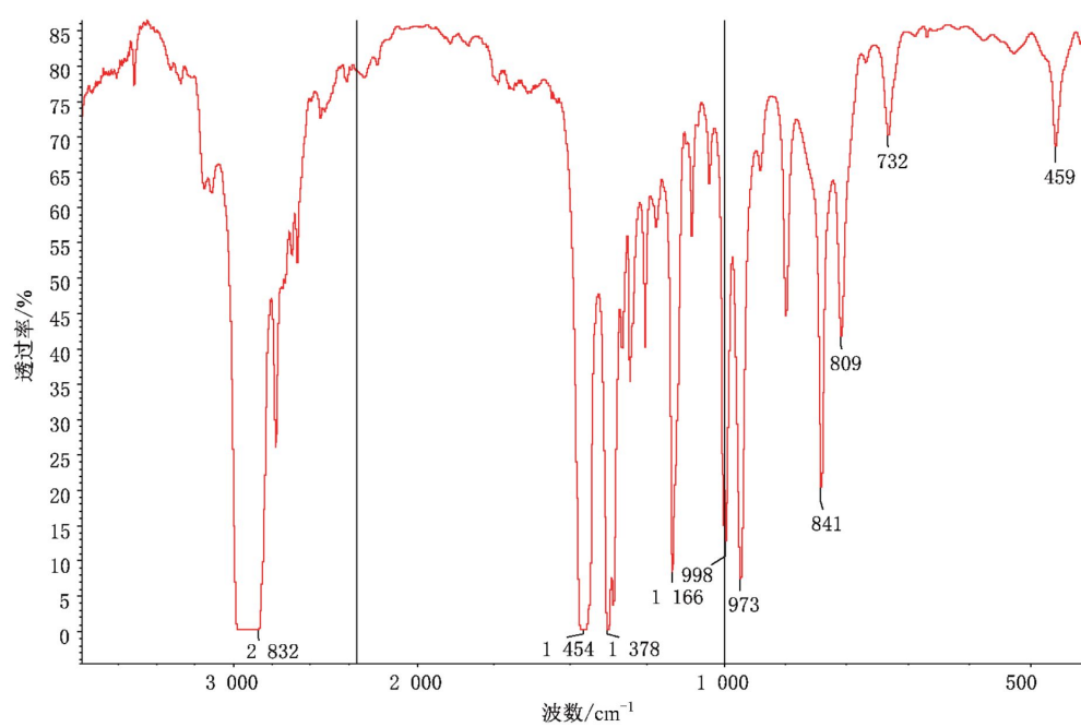
图 A.3 典型丙烯无规共聚物(PP-R)参考透射红外光谱图
