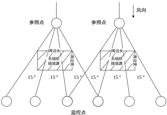
图D.4 多个无组织排放源监测采样点位示意图
