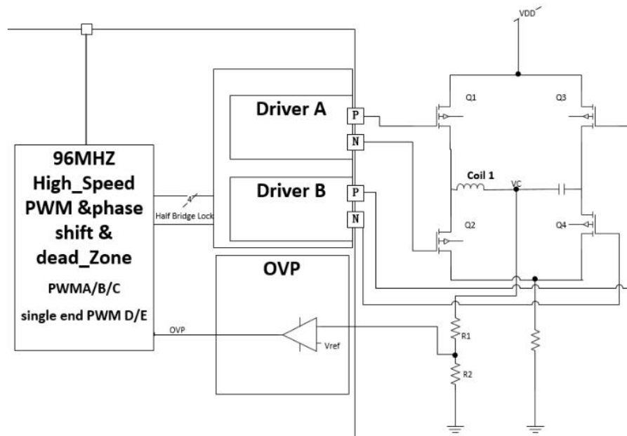
硬件保护电路框图
