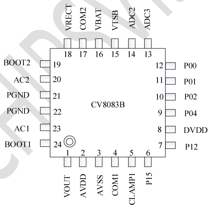
CV8083B引脚图
