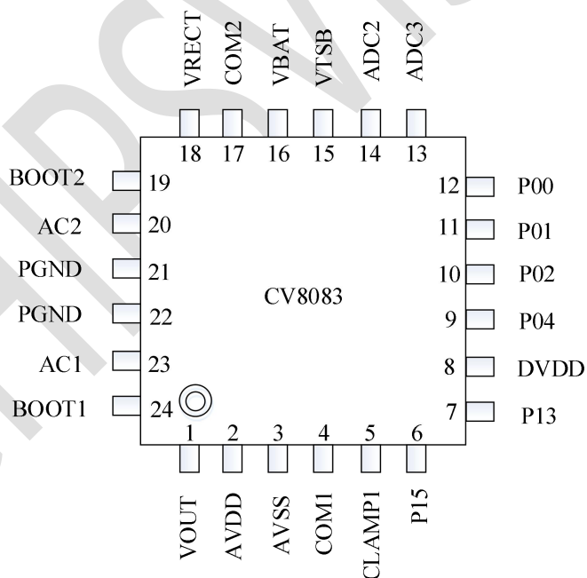
图3 CV8083引脚图
