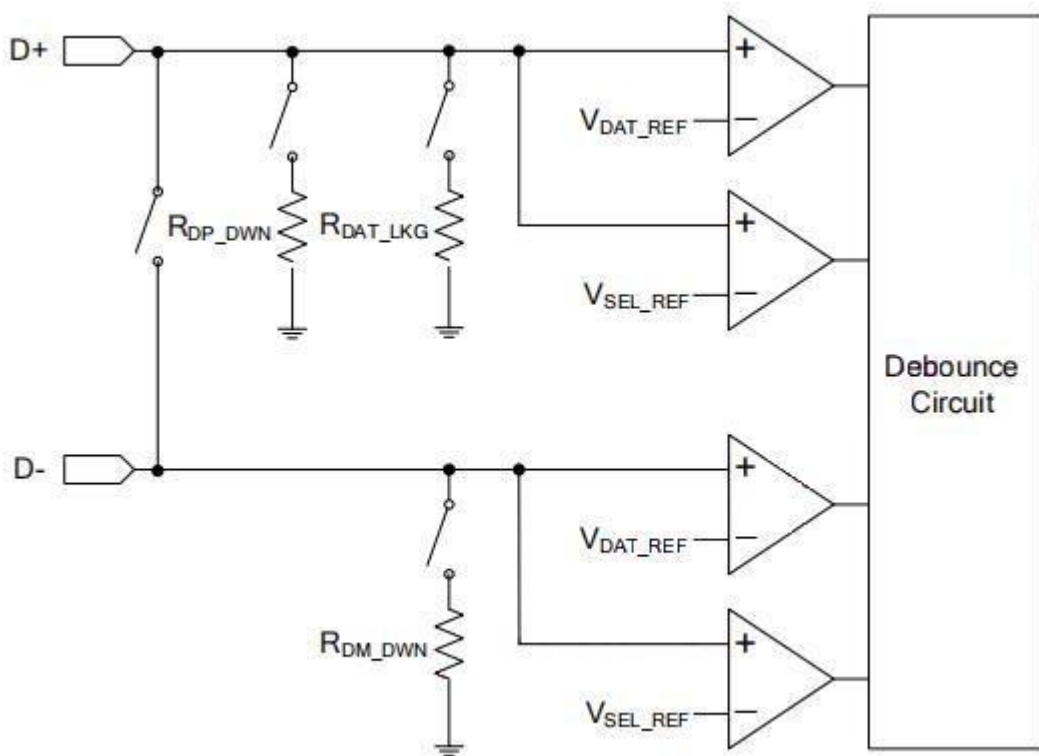
图3.2.3 USB 接口 D+, D- 内部线路示意图
