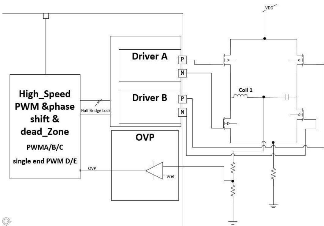
图3.8.1硬件保护电路框图
