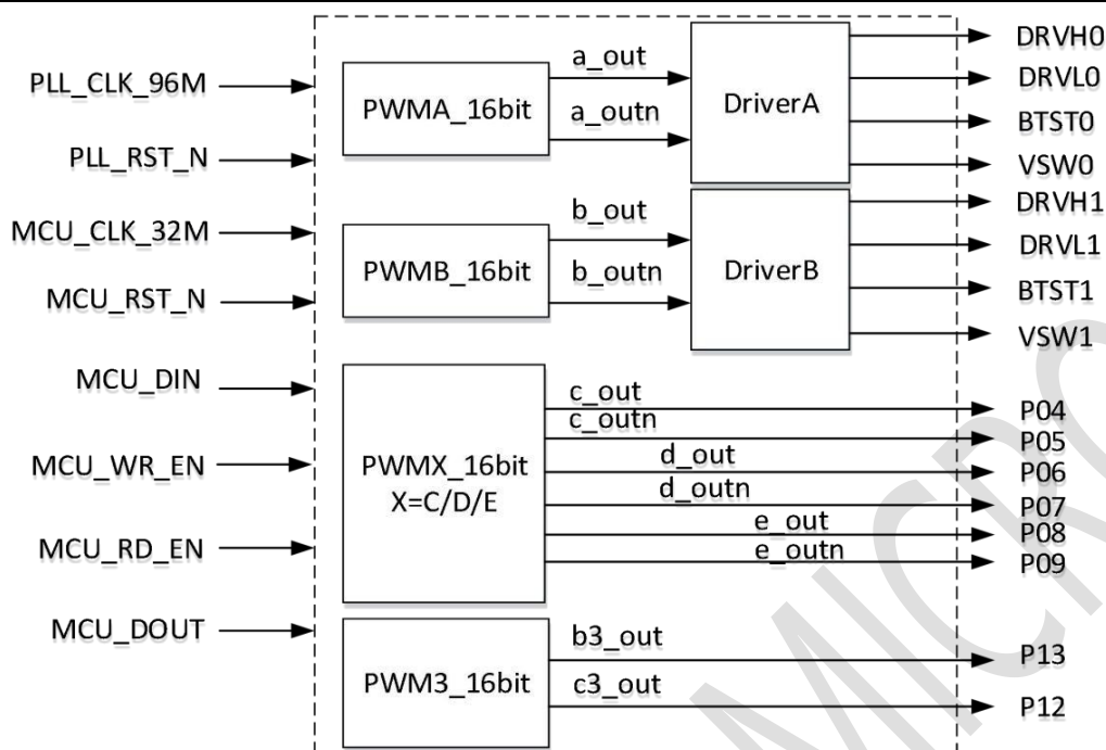
图3.5.1 全桥控制PWM图
