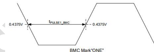
图 4. 4. 2a BMC 时间图
