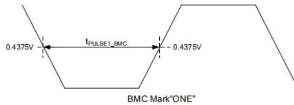
图 8.4.2a BMC 时间图
