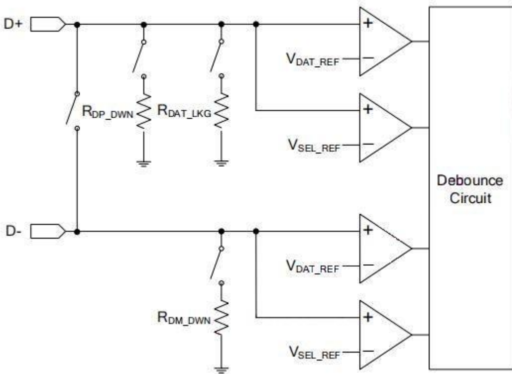
图7.2.3 USB 接口 D+, D- 内部线路示意图
