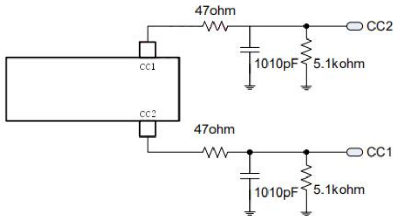
图 8.4.2b BMC 发射“1”讯号脉宽之测试电路
