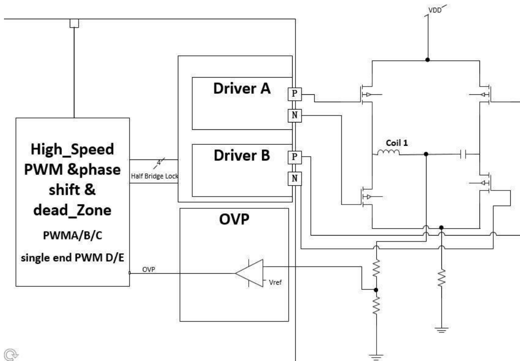
图7.8.1硬件保护电路框图
