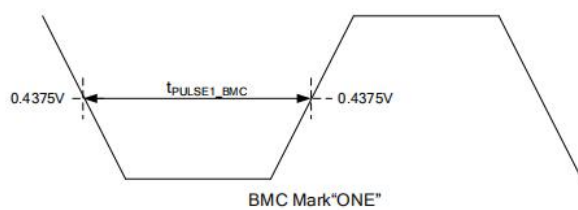
图 4.4.2a BMC 时间图
