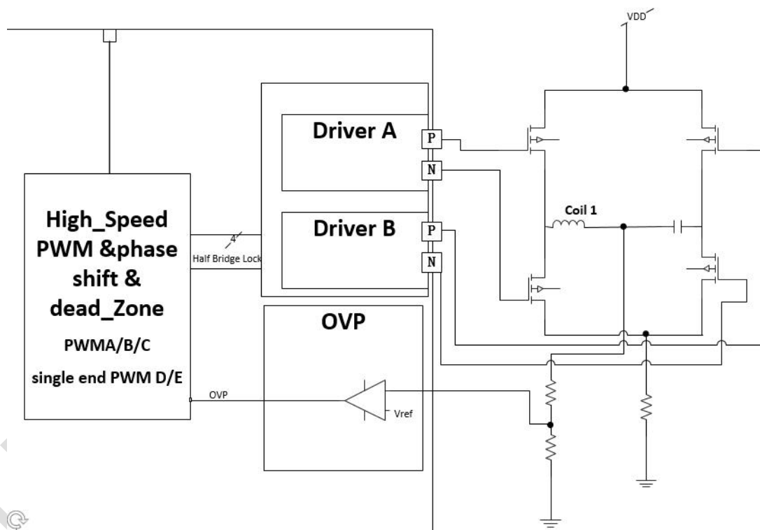
图3.6.1 硬件保护电路框图
