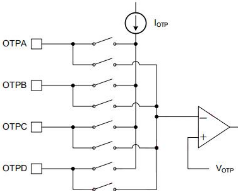
图3.8.3 外接温度检测元件示意图
