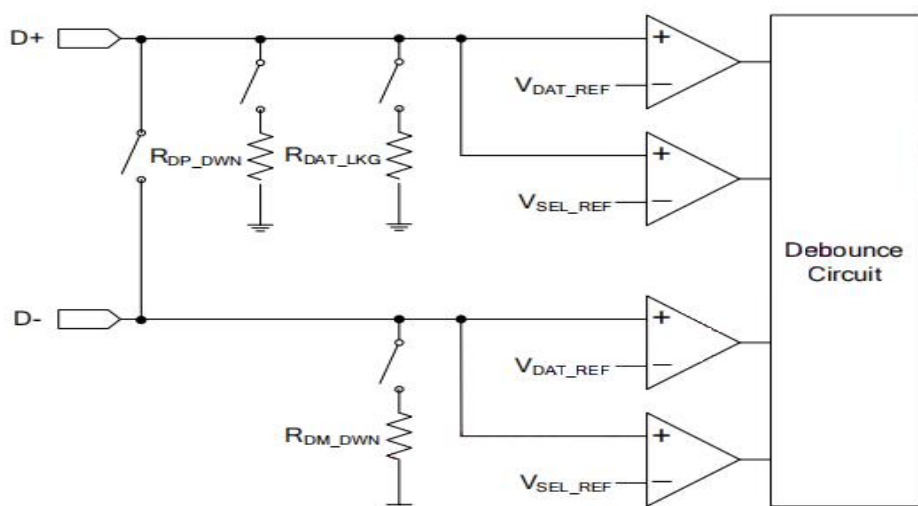
图3.2.3 USB 接口 D+, D- 内部线路示意图
