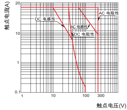
RKL1CO 最大负载通断曲线
