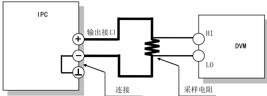
图 5-5 电流校准连接
