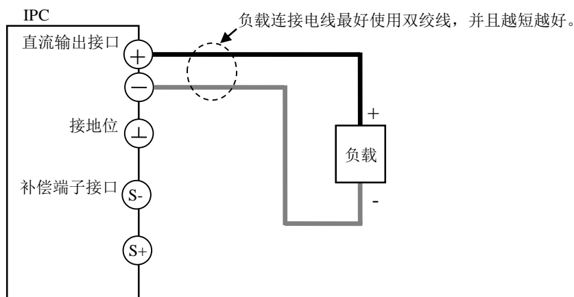
图 3-2 本地电压补偿模式
