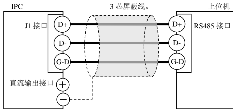
图 5-3 RS485 连接示意图
