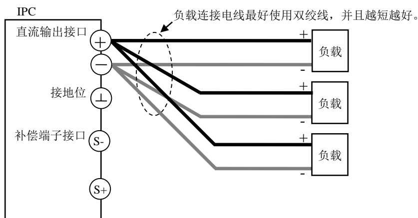
图 3-4 本地电压补偿模式下连接多个负载
