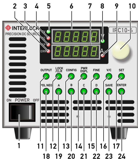
图 2-1 IPC 系列前面板
