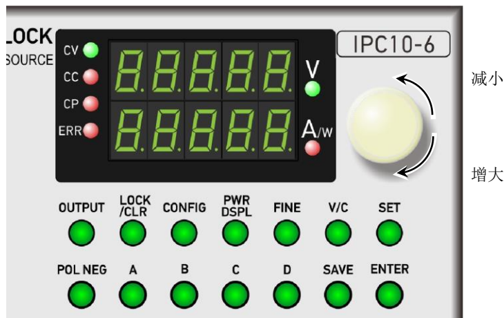
图 4-1 操作面板说明
