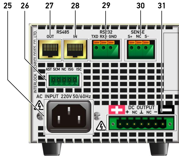
图 2-2 IPC 系列后面板
