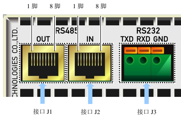
图 5-1 远程控制接口
