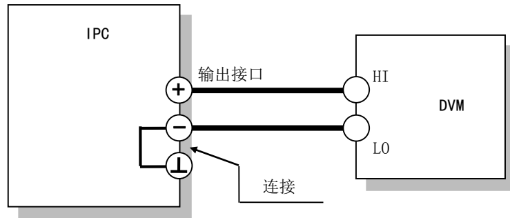
图 5-4 电压校准连接
