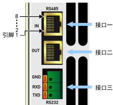
图 5-1 IPMP 系列远程控制接口
