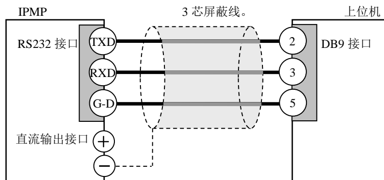
图 5-2 RS232 接口连接示意图
