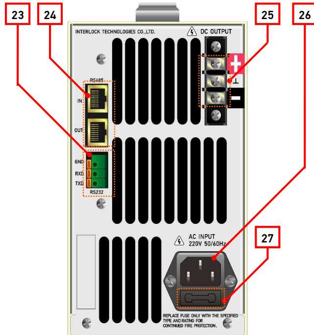
图 2-3 IPMP 系列后面板
