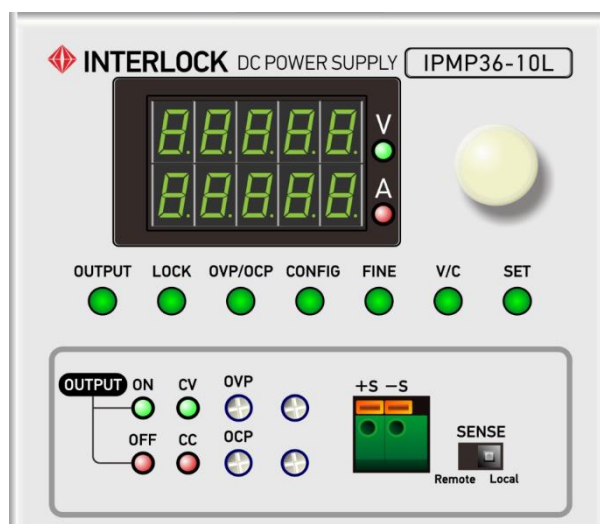
图 4-1 操作面板说明
