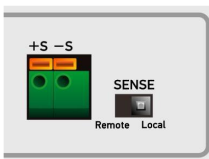
图 3-8 电压补偿端子
