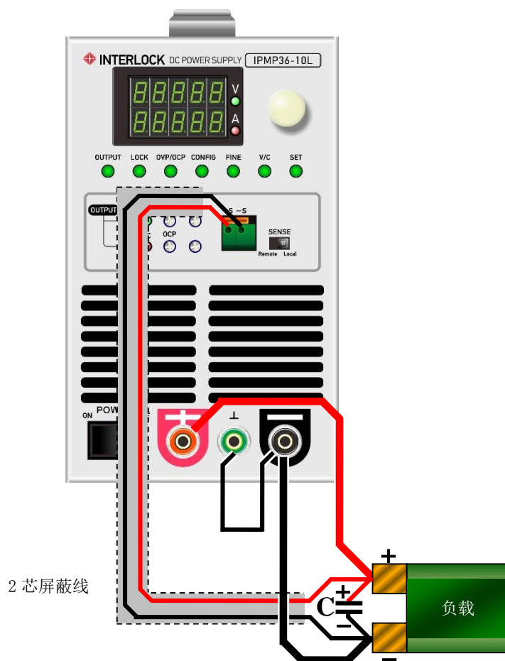
图 3-9 远端电压补偿接线图
