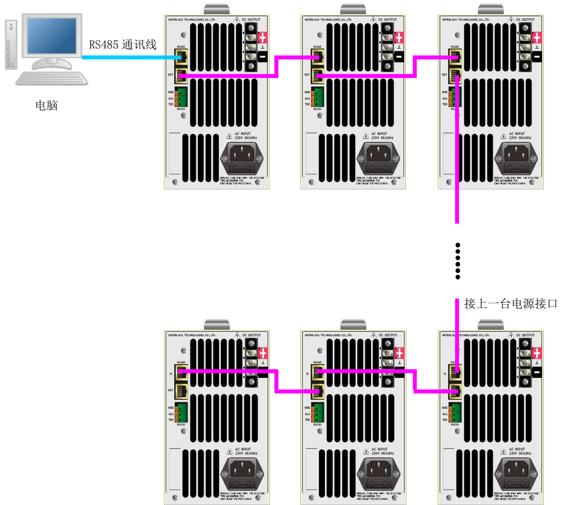
图 5-5 多台 IPMP 联网接线图
