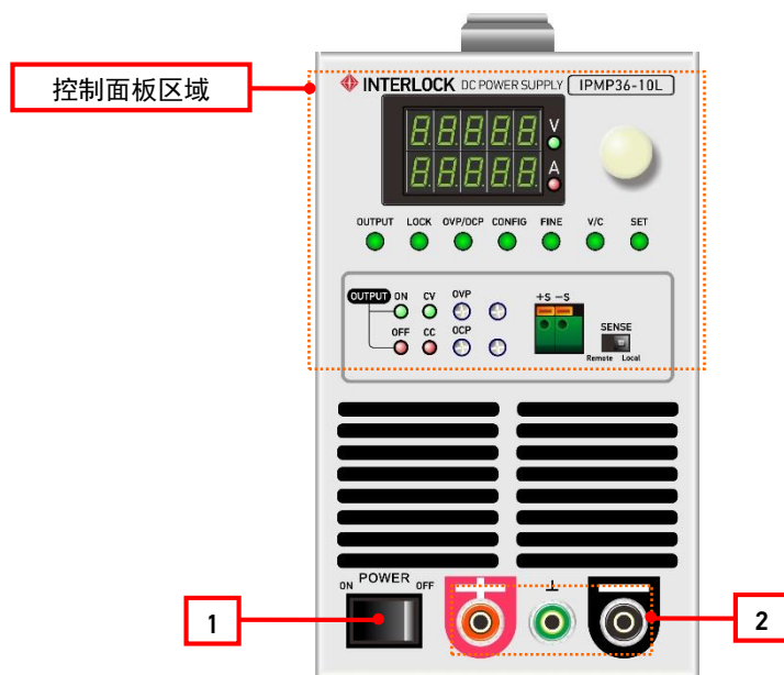
图 2-1 IPMP 系列前面板
