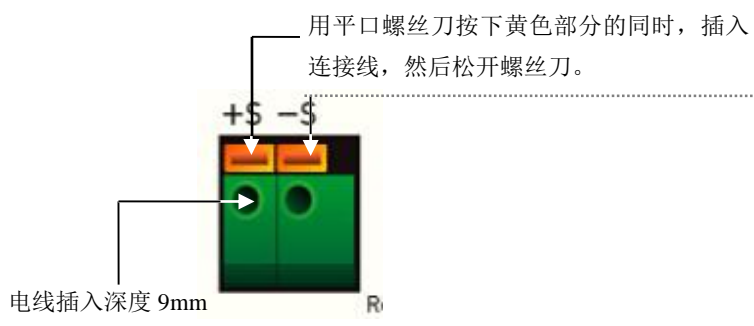
图 3-10 IPMP 系列远端补偿接口
