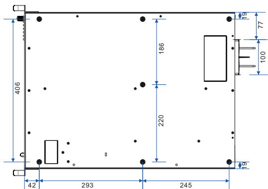
IPX-S系列 2~5kW 低压大电流尺寸 a示意图
