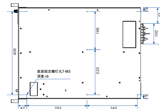
IPX-S系列 15kW 中高压小电流尺寸 f示意图
