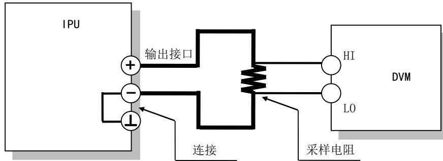
图 4-10 电流校准连接
