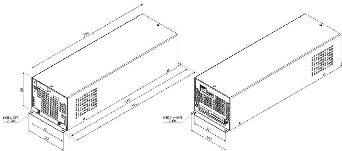
图 1-2 IPU 系列无显示模块
