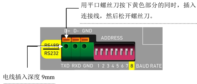
图 4-8 IPU 系列远程控制接口
