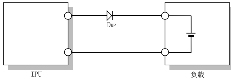
图 3-4 储能负载的连接方法
