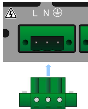
图 4-1 IPU 系列交流输入接口模块连接
