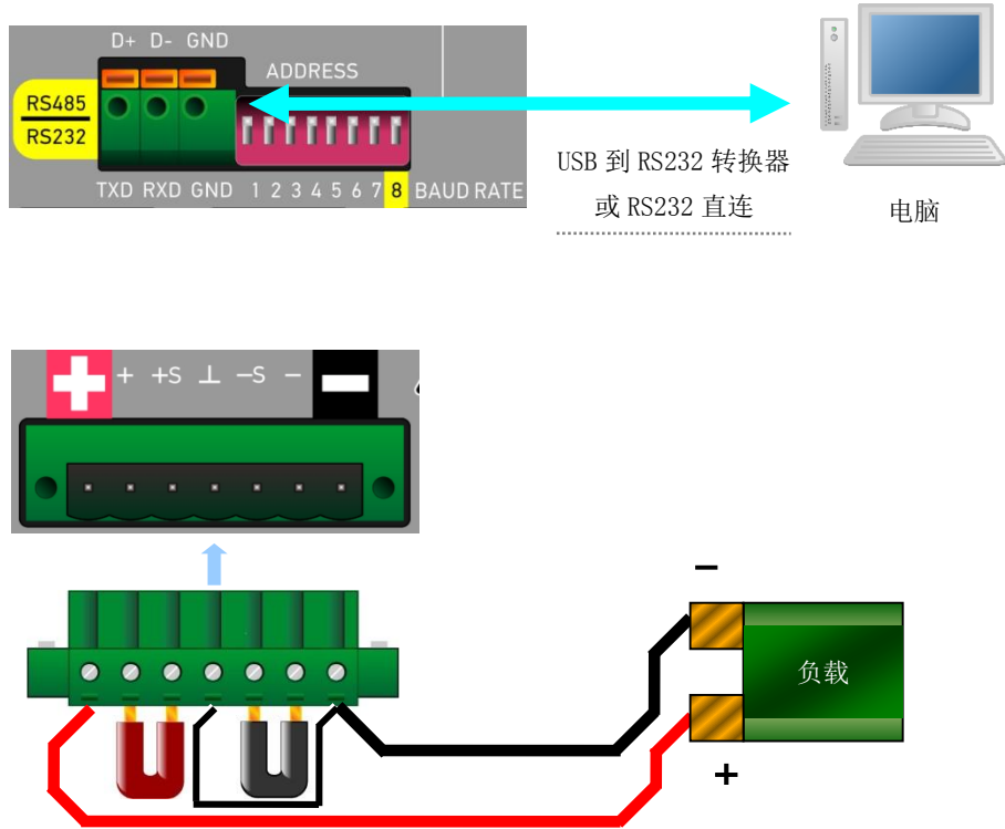
图 4-7 IPU 系列 RS232 接口连接图
