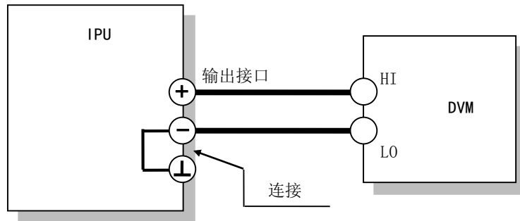
图 4-9 电压校准连接
