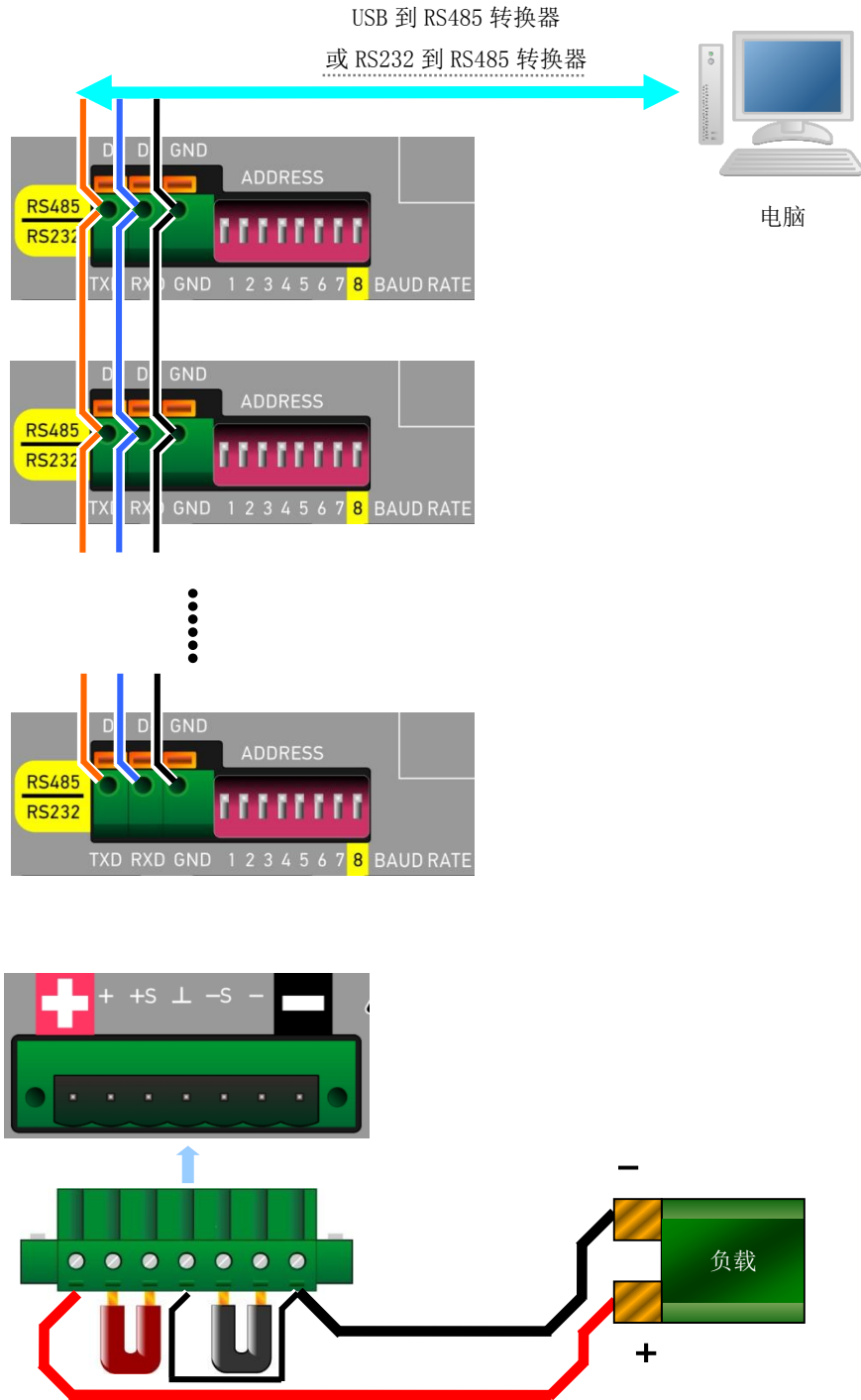
图 4-5 IPU 通过 RS485 接口多台联网接线图
