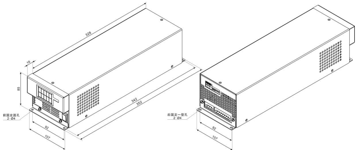
图 1-1 IPU 系列选配显示模块
