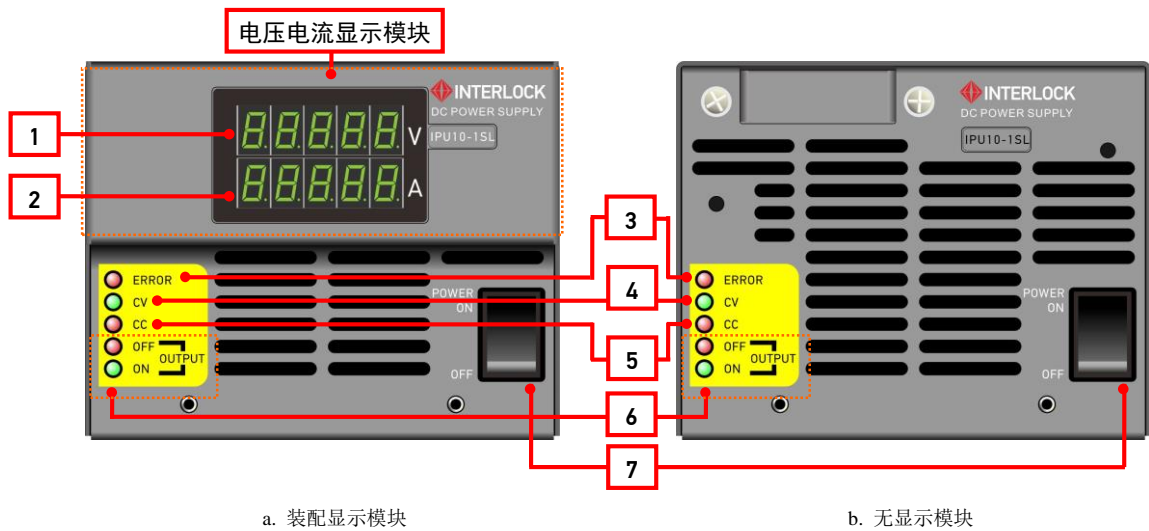
图 2-1 IPU 系列前面板
