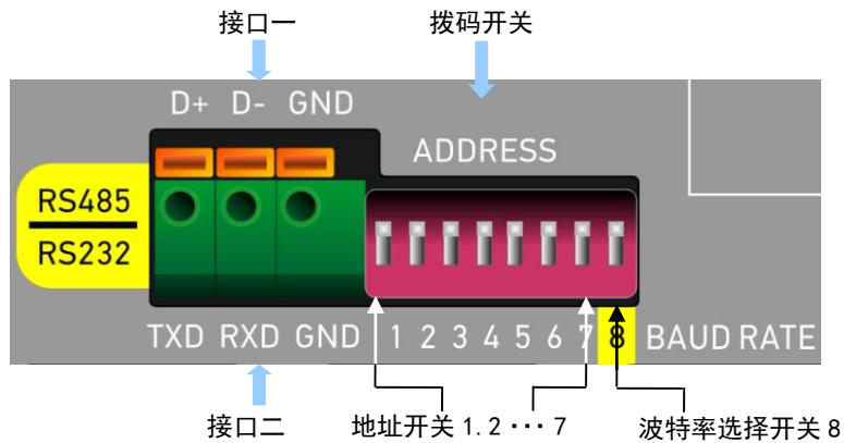
图 4-3 IPU 系列远程控制接口
