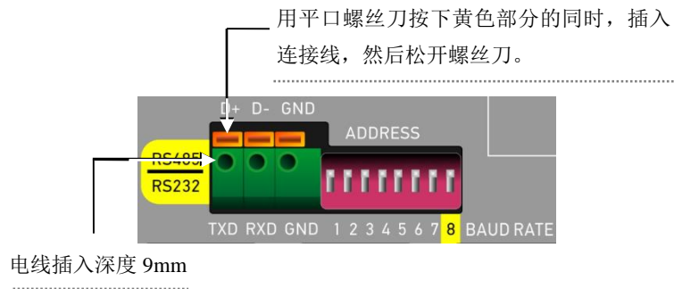
图 4-6 IPU 系列远程控制接口
