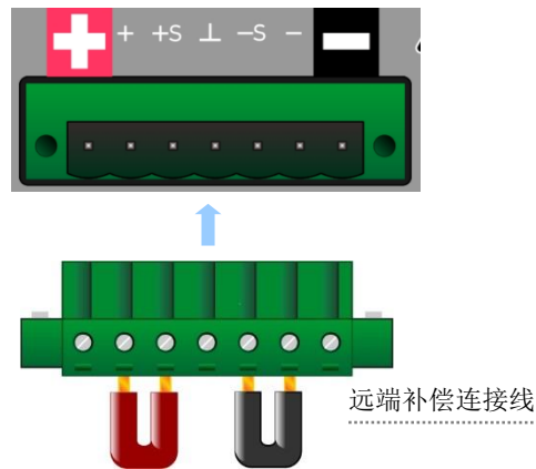
图 4-2 IPU 系列交流输入接口模块连接
