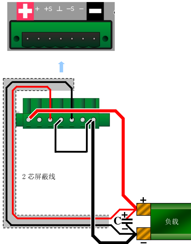
图 6-1 远端补偿接线图
