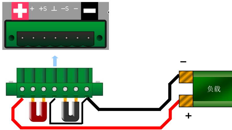
图 4-4 IPU 系列 RS485 接口连接图
