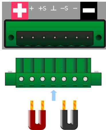
图 6-2 远端补偿连接线图
