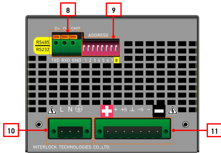
图 2-2 IPU 系列后面板
