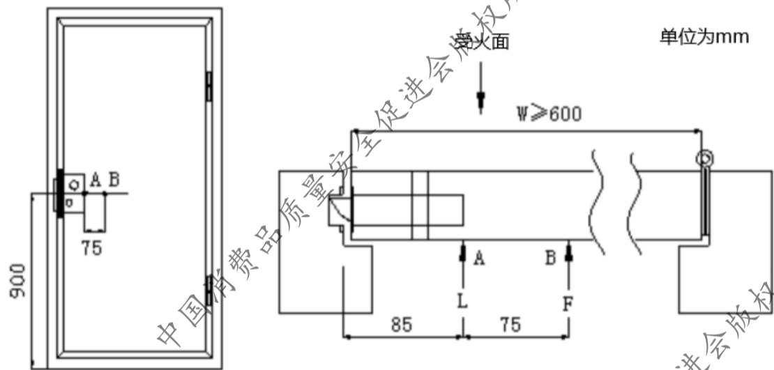
图2 试件安装示意图
