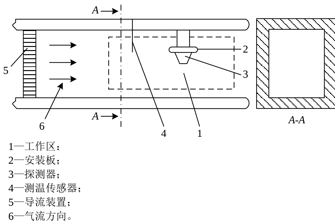
图 A.1 标准温箱工作区域示意图
