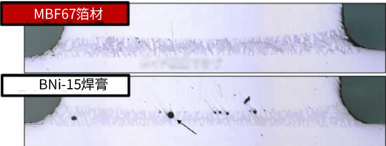
不锈钢SUS316接合后的断面 (本公司比较)
