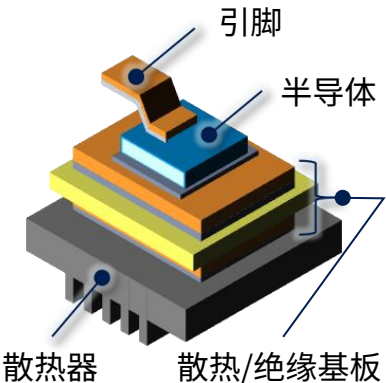
功率模块
