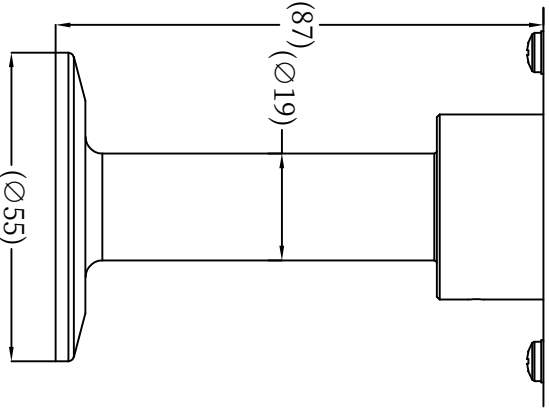
KF40屏蔽加强型
