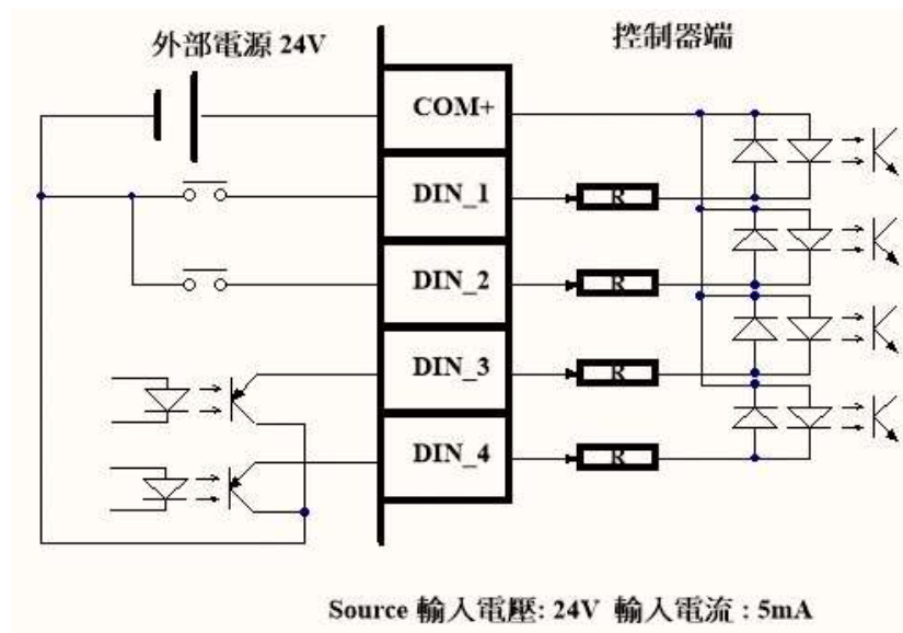
图 5-2 DIN 的 Source 接法
