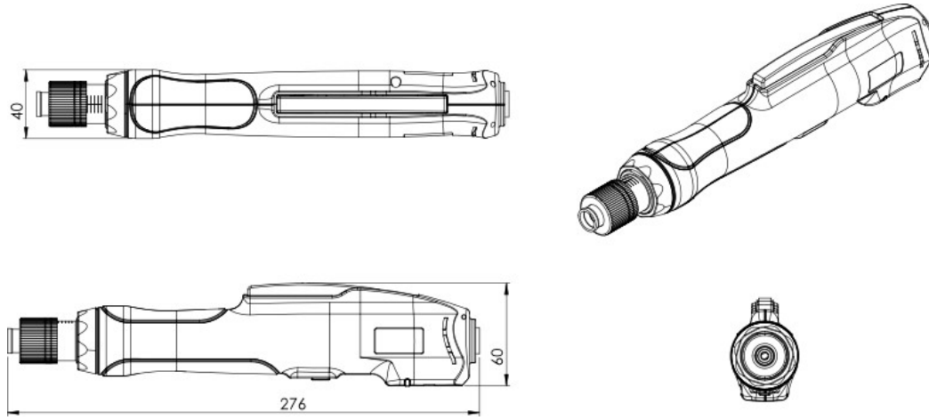
图 3-2 工具外观(单位: mm)
