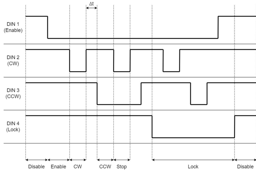
图 5-5 IO-DIN 控制时序图
