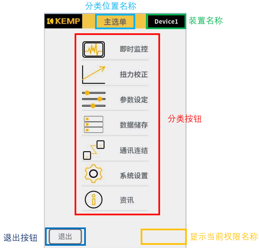
图 4-2 主画面
