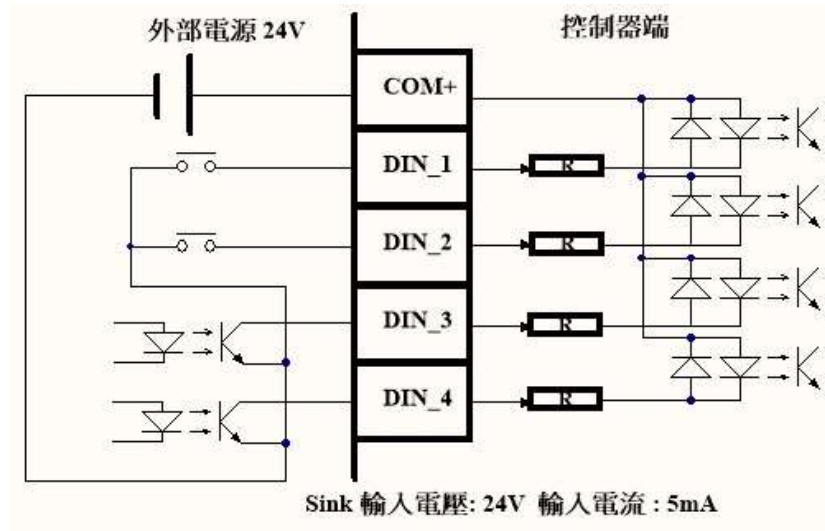
图 5-1 DIN 的 Sink 接法
