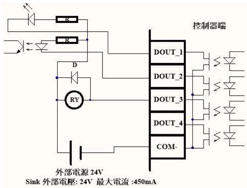
图 5-3 DOUT 的 Sink 接法
