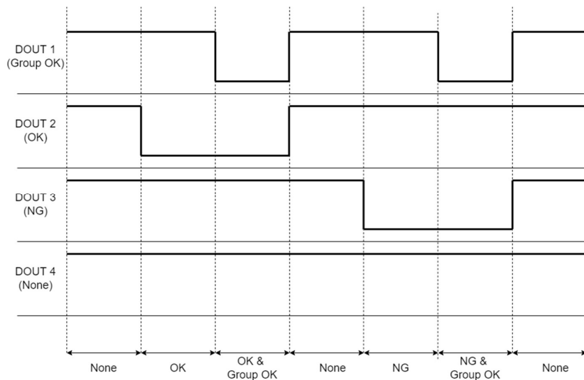
图 5-6 IO-DOUT 控制时序图
