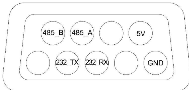
图 3-5 DB-9 连接引脚定义
