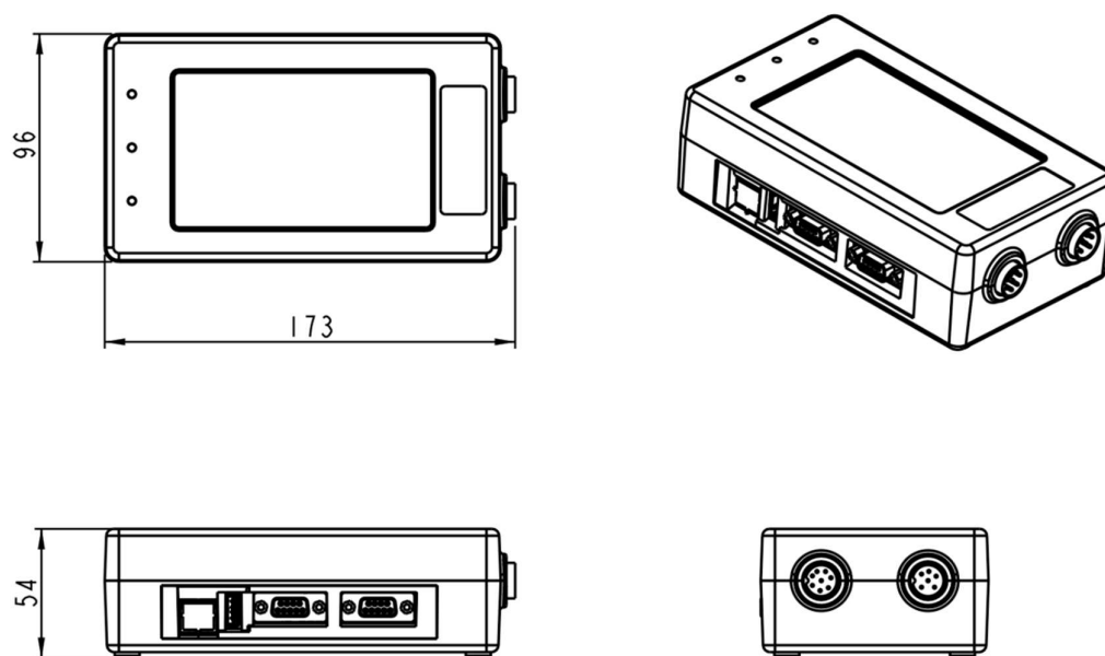
图 3-3 控制盒外观 (单位: mm)
