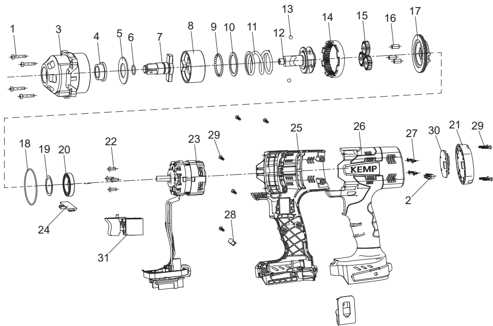
零件爆炸图 CBI-AD4200
