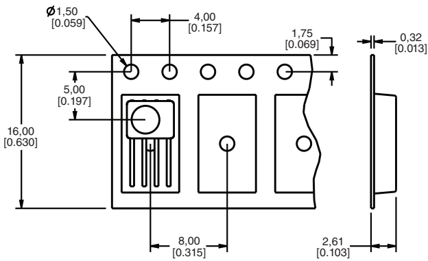
卷带包装 1
