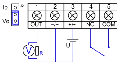
0~10V 输出
