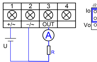
4~20mA 输出
