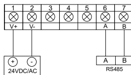
RS485输出
