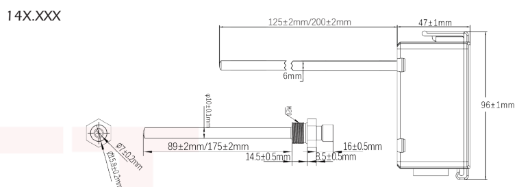
水管型 温度传感器 / 变送器
