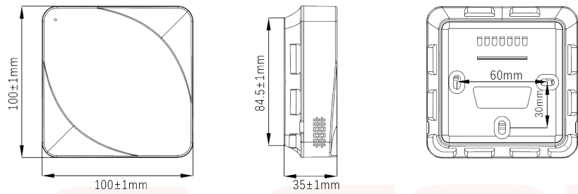
AQ12.XX/AQT12.XX
