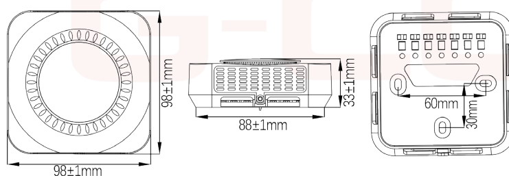
壁挂型 多参变送器
