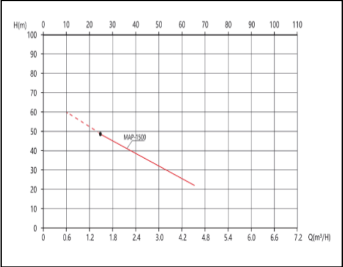
水泵性能
