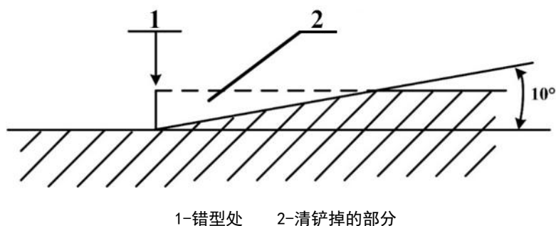
图 1 错型处清铲成 10^\circ 的斜坡面
