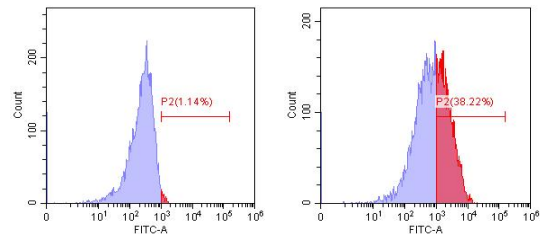
图 1. 应用本产品制备的靶向人 CD22 CAR-T 细胞 CAR 表达水平约 37%。分别取 2 \times 10^5 的 T 细胞和靶向人 CD22 CAR-T 细胞，用 2μl FITC-Labeled Human CD22 Protein 进行染色。图左：T 细胞，图右：靶向人 CD22 CAR-T 细胞。
