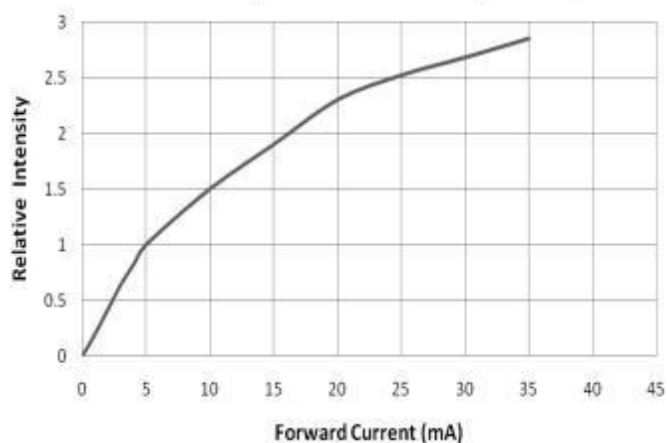
相对光强与电流特性曲线 Relative Intensity VS. Forward Current ( T_a=25^\circ\text{C} )
