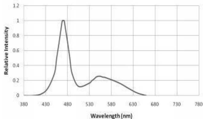
光谱分布特性曲线 Spectrum Distribution ( T_a=25^\circ\text{C} )
