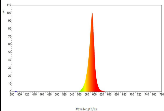
Spectrum Distribution / 相对光普能量百分比曲线图
