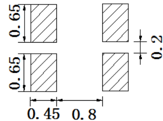
建议焊盘尺寸图:
