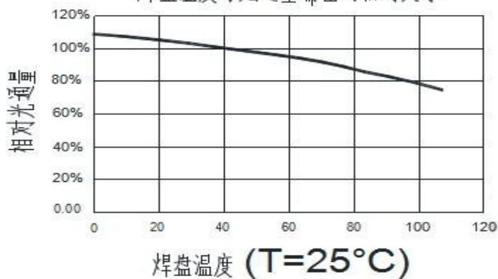
焊盘温度与光通量输出的相对关系
