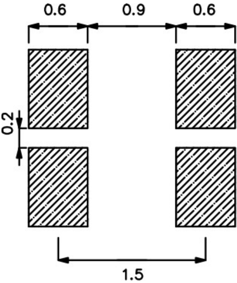
焊盘及焊锡脚示意图
