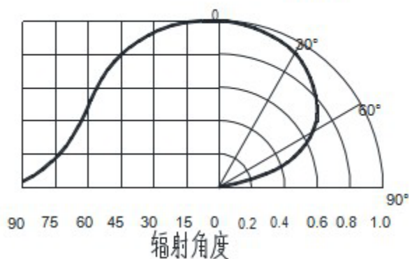
典型的辐射方向图 120°
