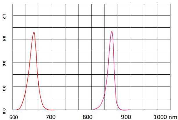
Spectrum Distribution / 相对光谱能量百分比曲线图
