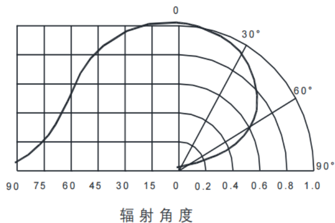
典型的辐射方向图 120°
