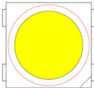
OK(吸嘴内径大于灯珠发光区)
