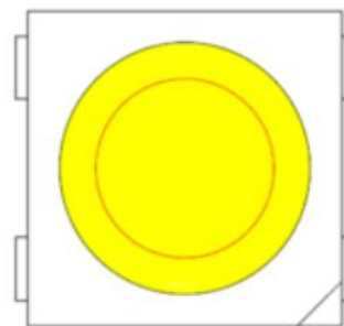
NG (吸嘴内径小于灯珠发光区)
