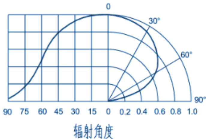
典型的辐射方向图 120°
