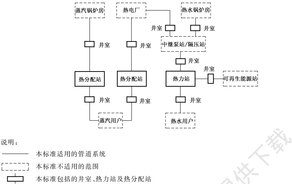
图 2 本标准适用的热力管道系统范围
