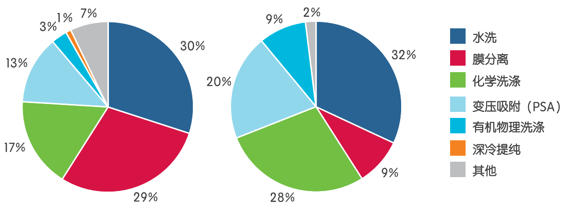
图12：沼气提纯技术市场份额，根据运行工厂数量确定
