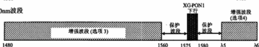
图5 波长分配图示
