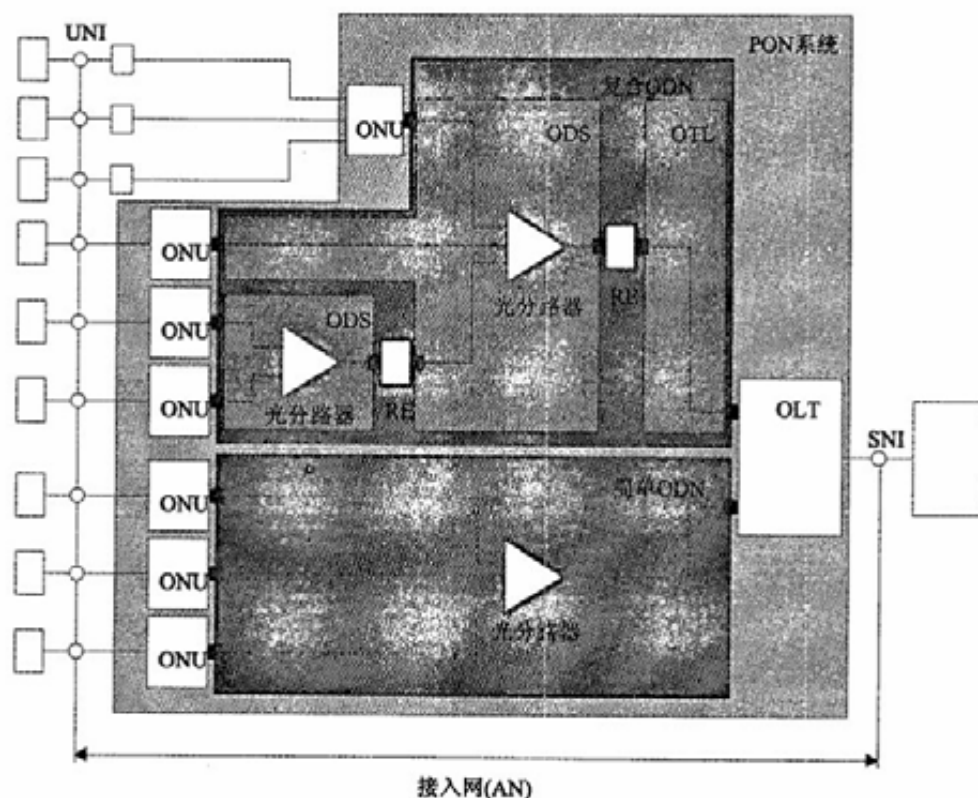
图2 XG-PON 网络参考结构
