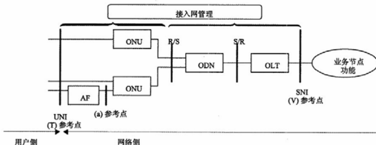
图1 XG-PON 参考配置
