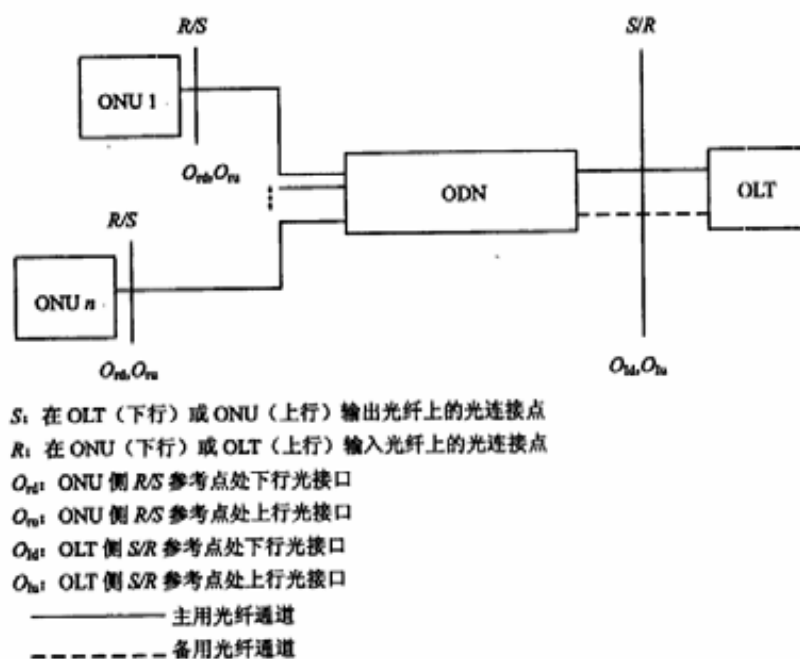
图1 ODN 通用物理配置
