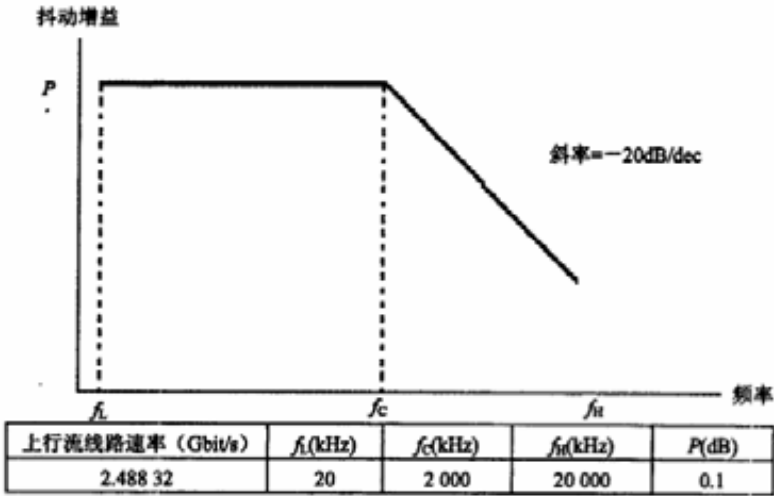
图5 ONU 抖动转移
