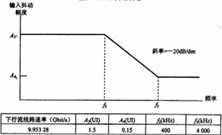
图6 正弦抖动模板的高频部分
