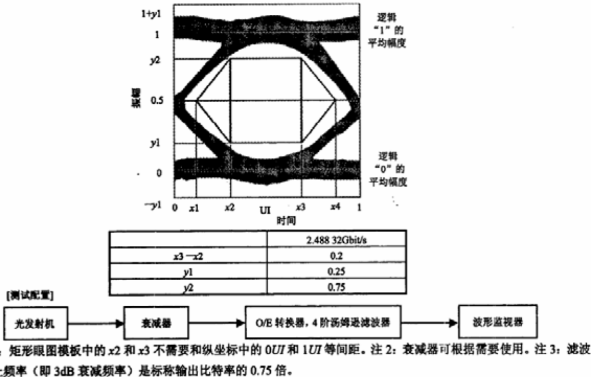
图4 ONU 发射机眼图模板
