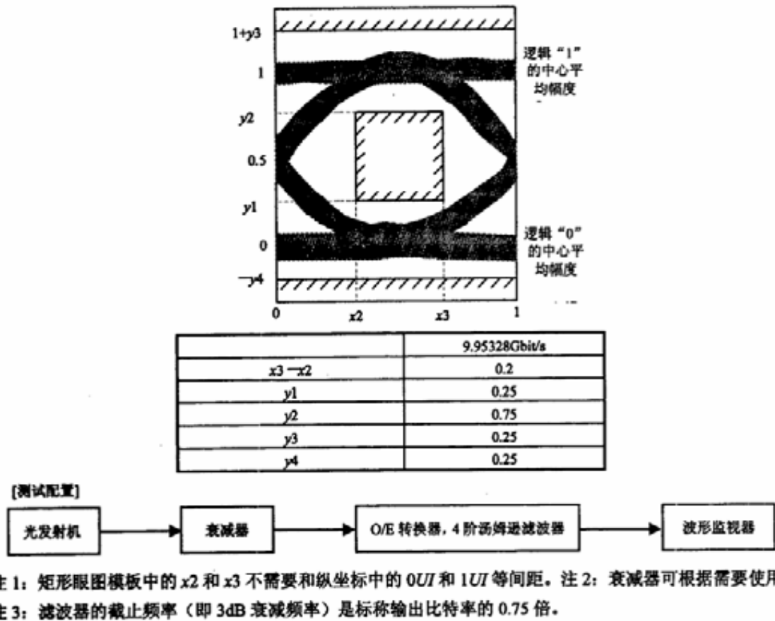
图3 OLT 发射机眼图模板
