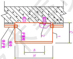
图1 明装方式
