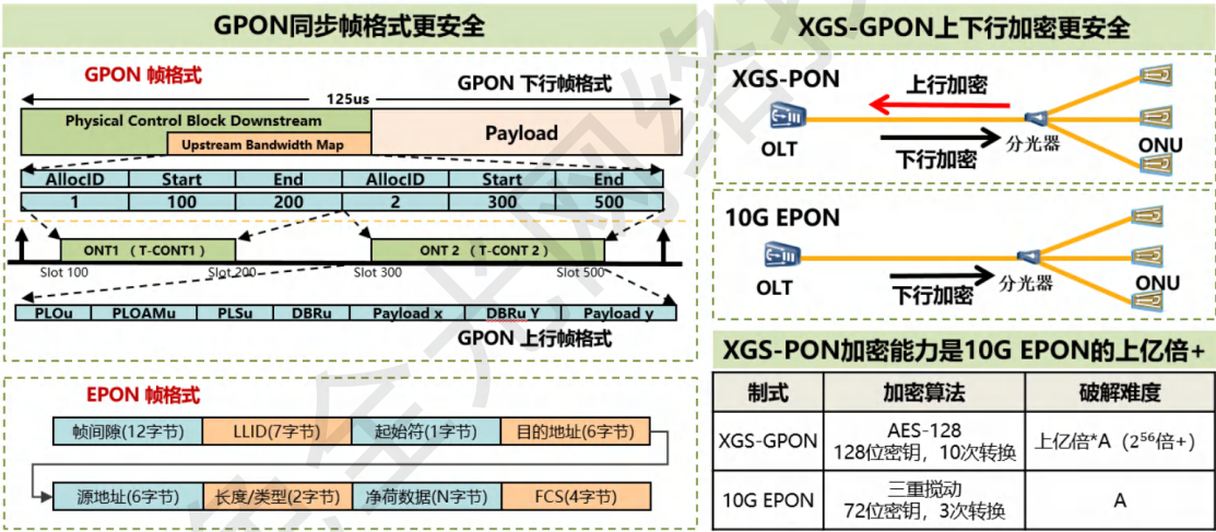
图 1-16 GPON/EPON 系列安全性比较
