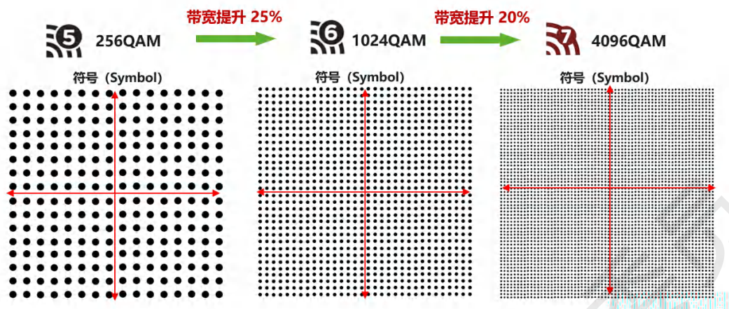
图 1-8 F5G 全光网 Wi-Fi 接入的编码方式
