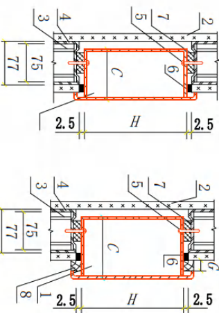
图1 方式 (1)
