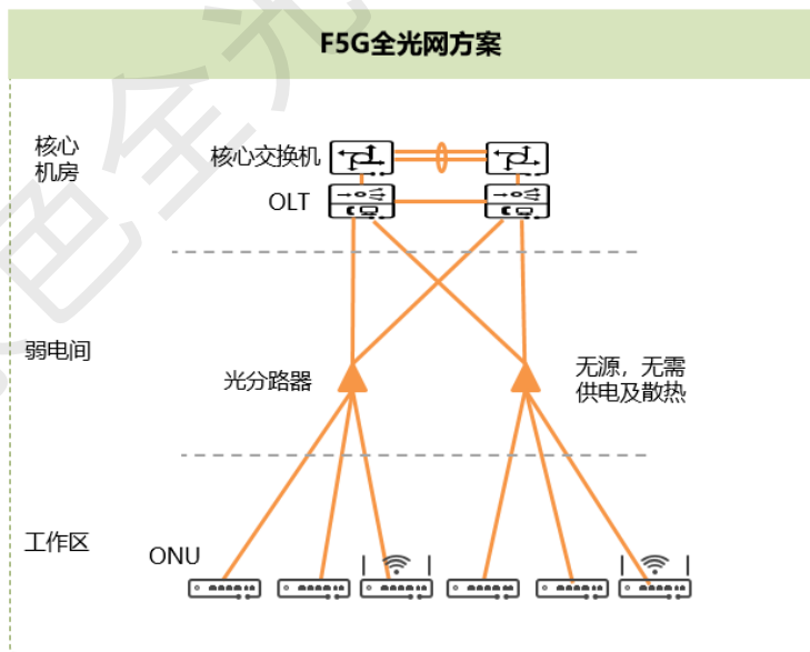
图 1-9 F5G 全光网简化网络
