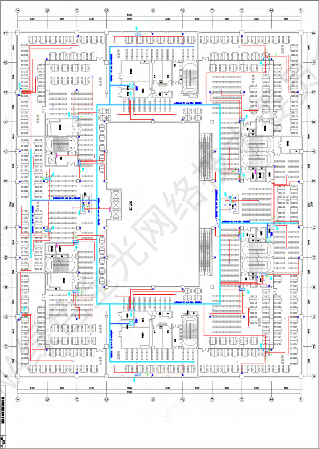
图书馆校园信息网平面图，详图请参见设计指南图集.dwg 文件
