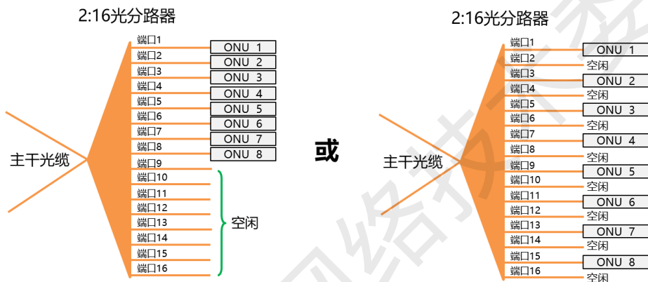
图 2-26 2:16 光分路器当作 2:8 使用
