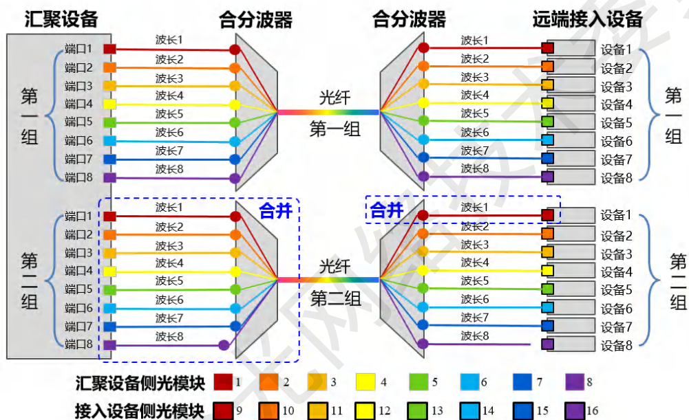
图 1-18 CWDM 方案技术原理示意图
