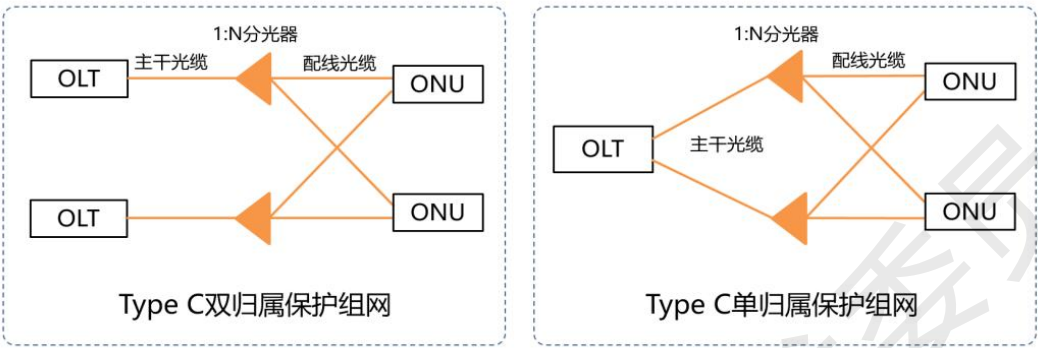
图 2-3：F5G 全光网 Type C 保护方式
