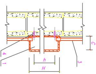
图2 明装安装方式
