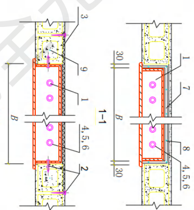
图1 安装方式 (1)
