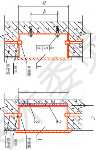
图1 暗装方式 (1)
