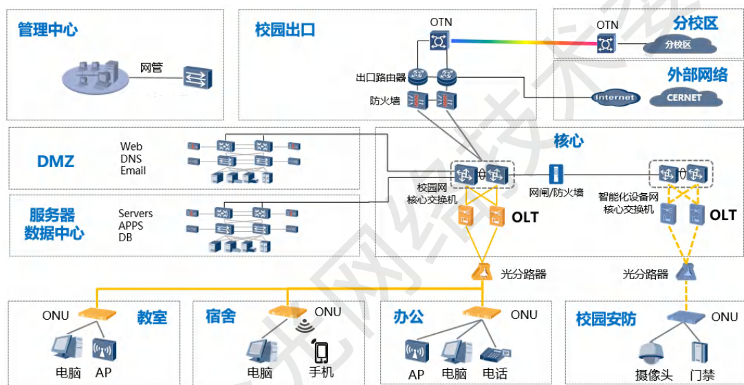
图 1-4 智慧教育 F5G 全光网网络架构
