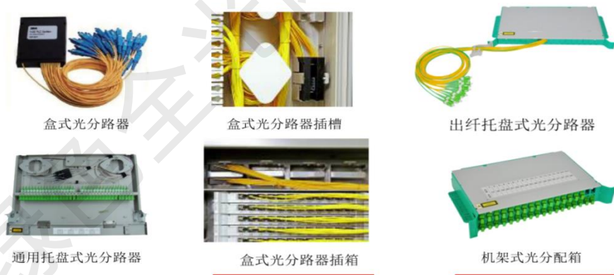
图 2-25 F5G 全光网光分路器的类型选择
