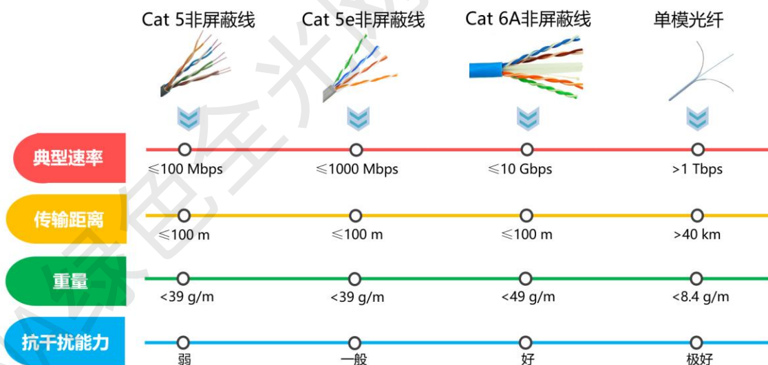
图 1-5 网线与光纤的传输性能/重量对比
