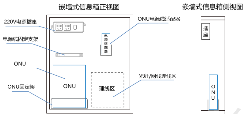
图 2-15 嵌墙式信息配线箱内部安装位置图（单台非 POE ONU）
