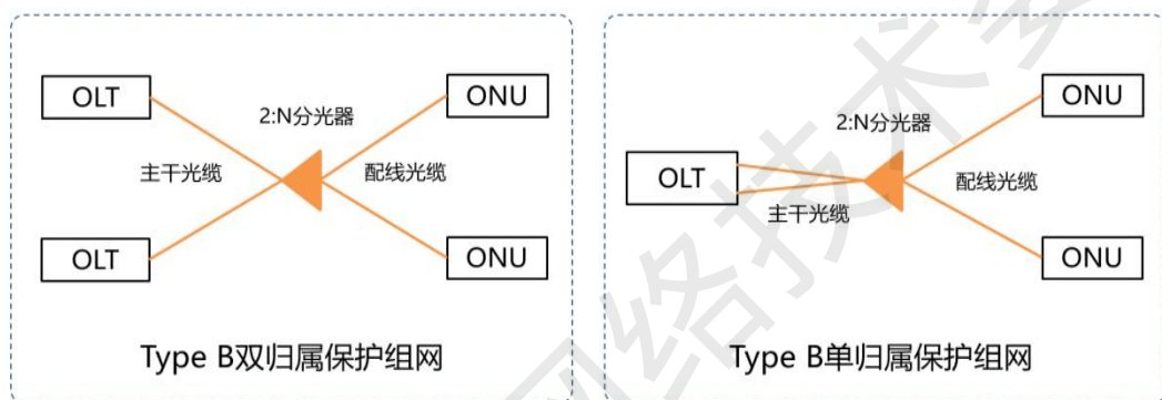
图 2-2：F5G 全光网 Type B 保护方式
