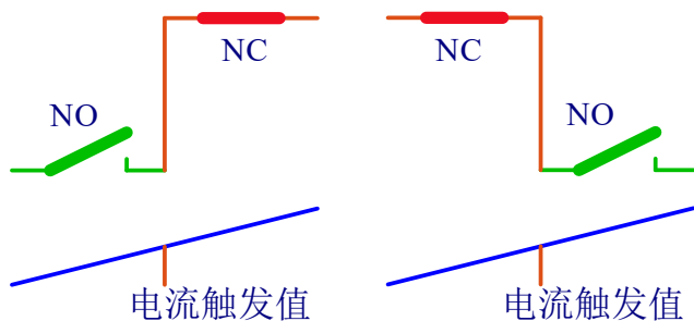
常开逻辑原理
