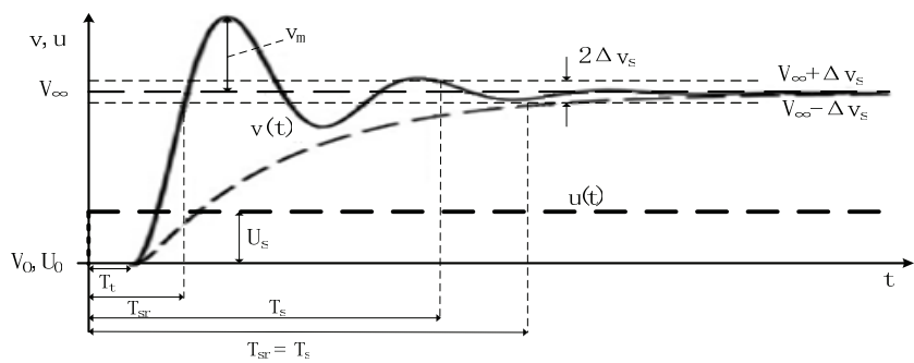
图1 阶跃响应
