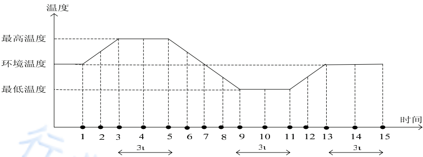
图 3 温度循环准确度试验
