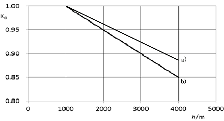
图 2 温升的海拔校正因数
